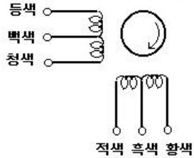
H-548 모터의 내부결선 및 회전방향
